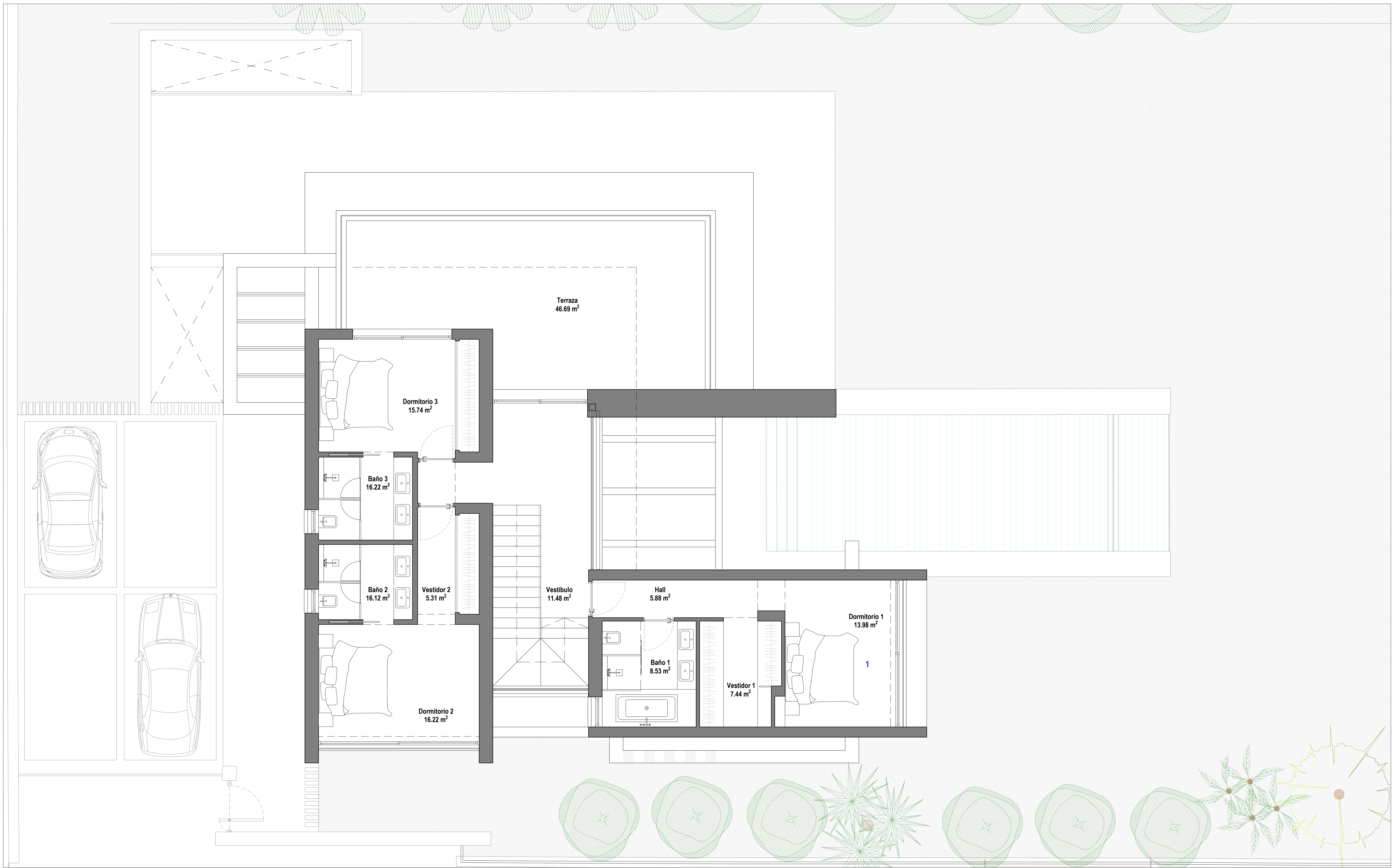
PLANTA PRIMERA_E:1.50
